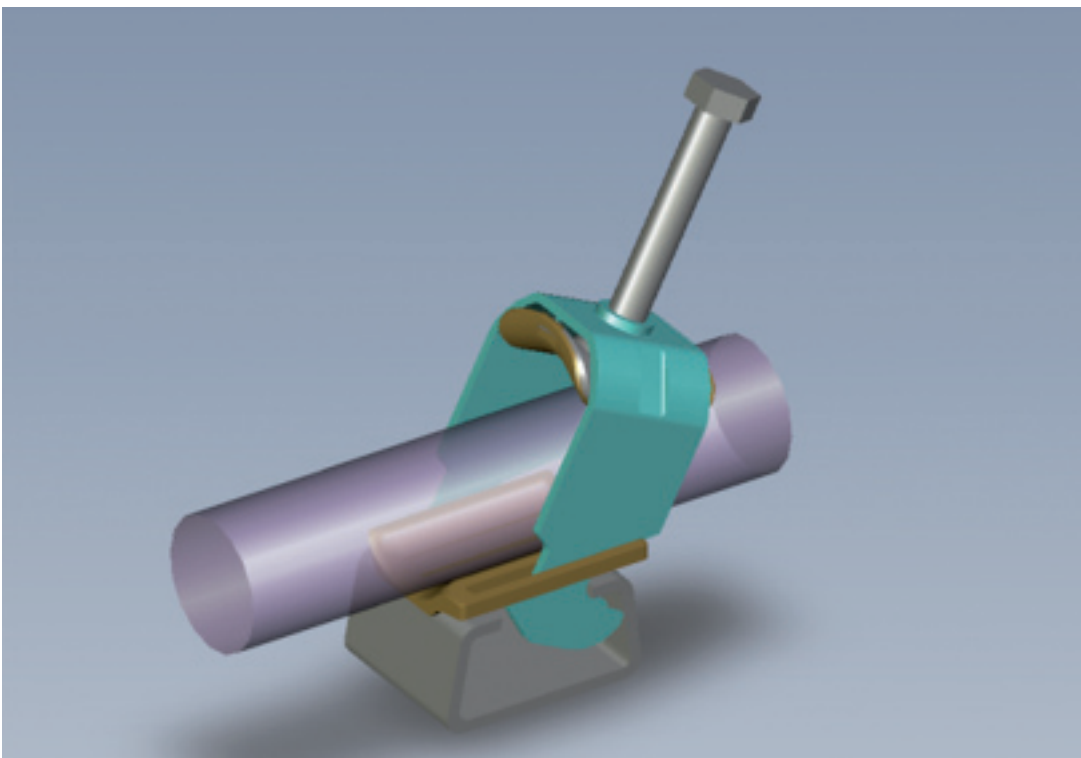
Bild 7: Neue Bügelshelle mit Simulation des Einhängens in die Halteschiene
